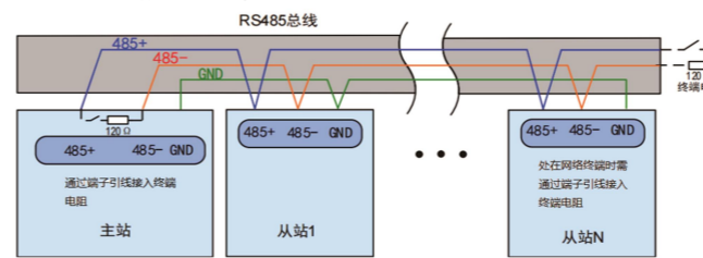
图 9 RS485 总线通信示意图
