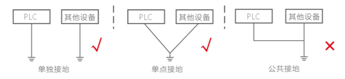
图 1 接地类型图
