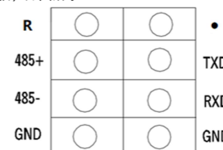
图 8 RS485 & RS232 通信端口示意图
