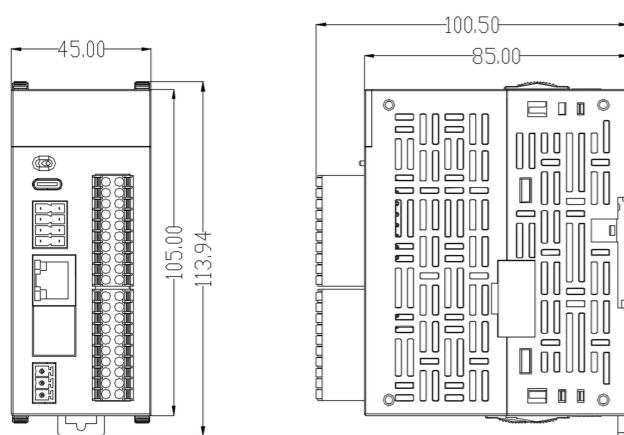
图 3 SC2-C 系列产品外观尺寸图 (单位: mm)
