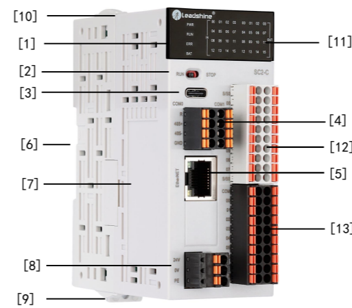
图 2 SC2-C32A4DS 产品外部接口
