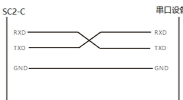
图 10 RS232 总线通信示意图
