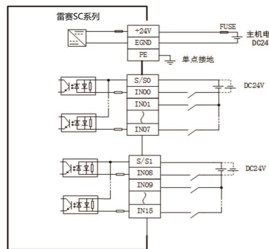
图 4 SC2-C 系列产品输入口等效电路
