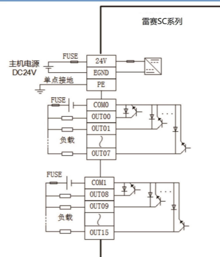
图 5 SC2-C 系列产品输出口等效电路
